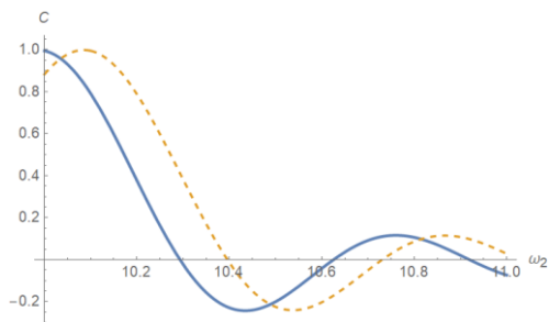
Рис. 2. Коэффициент корреляции гармонических сигналов в зависимости от \omega_2 . Значения параметров равны d_1 = 0 , d_2 = 0.1 , L = 10 , \omega_2 = 10 (сплошная кривая), \omega_2 = 10.1 (пунктирная кривая)
